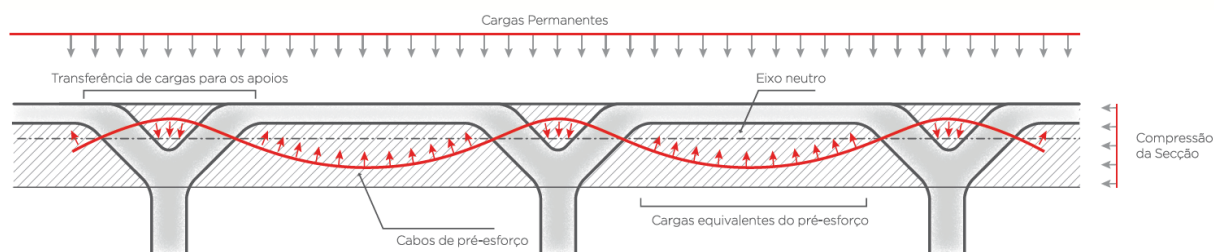
Figure 14 – Charges équivalentes de la précontrainte sur la dalle COBIAX CLS
