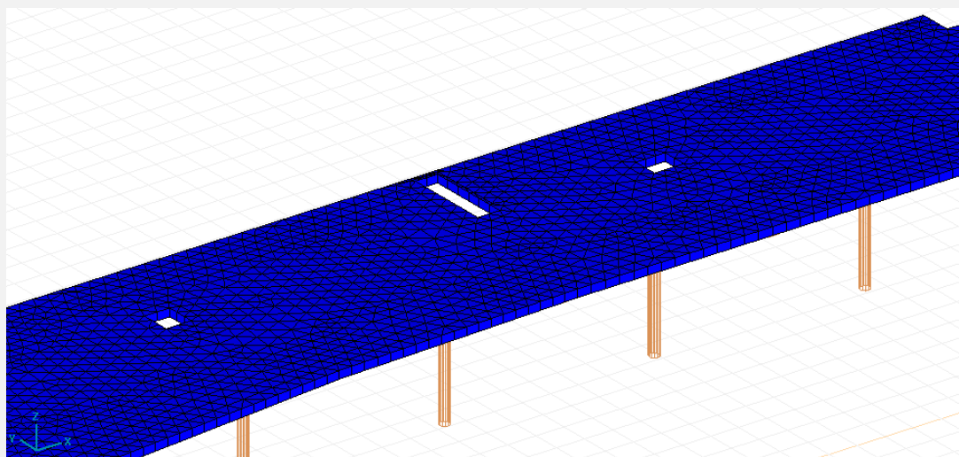
Modèle de calcul d'une dalle (visualisation 3D) contenant quelques ouvertures et supporté par des colonnes
