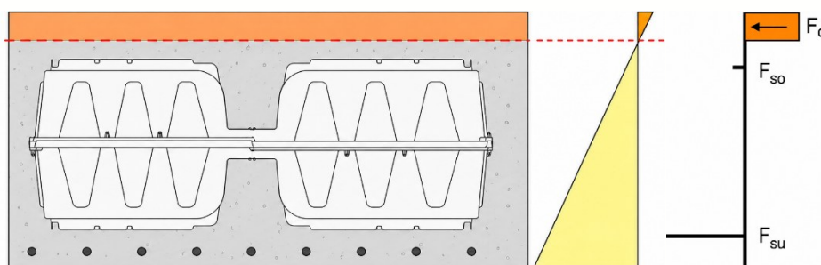
Figure 7 – Position de la ligne neutre au-dessus du vide dans la lame de compression.
