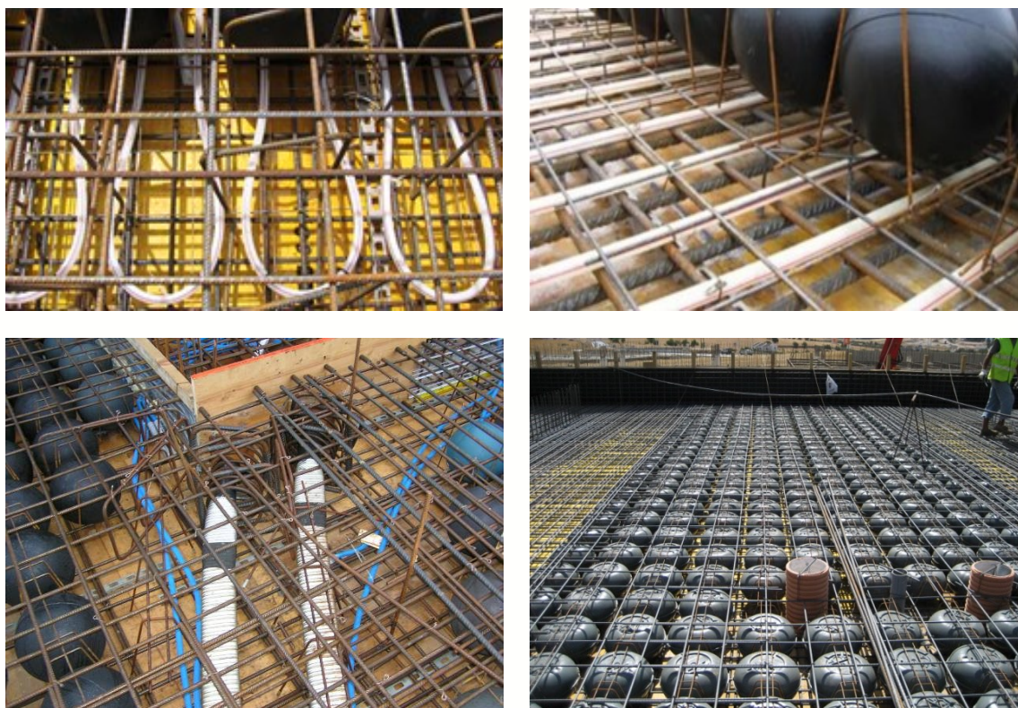
Figure 16 - Exemples d'installations diverses et systèmes de post-contrainte dans une dalle COBIAX CLS
