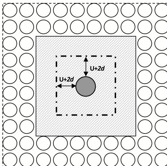
Figure 10 – Zone pleine pour le poinçonnement
