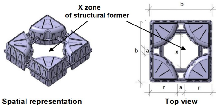
Figure 8 – Définition de la zone X
