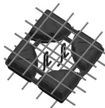
Figure 9 – Position des omégas à l'intérieur de la Zone X
