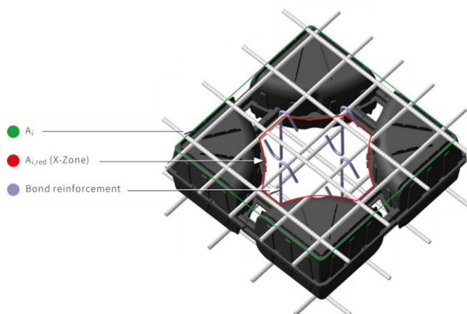
Figure 11 – Exemple de renforcement dans la zone X d'une dalle Cobiax CLS
