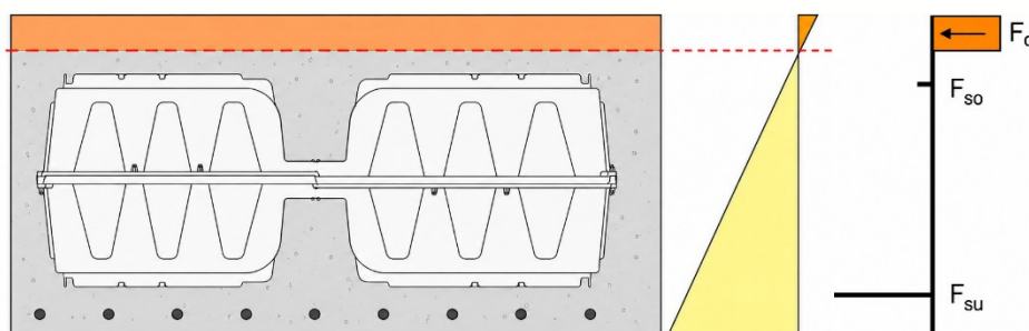
Figura 7 – Posición de la línea neutra por encima del hueco en la lámina de compresión.
