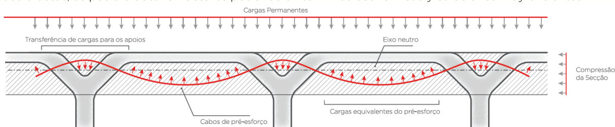
Figura 14 – Cargas Equivalentes del Postesado en el forjado COBIAX CLS
