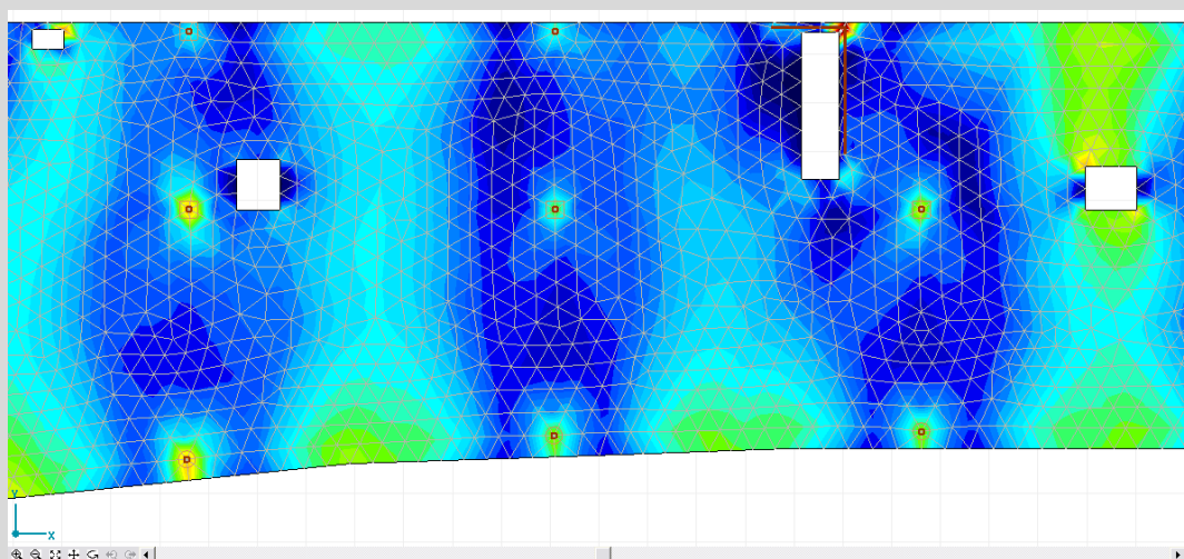
Distribución de los esfuerzos en estados límite últimos
