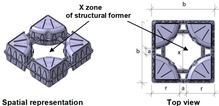
Figura 8 – Definición de la zona X
