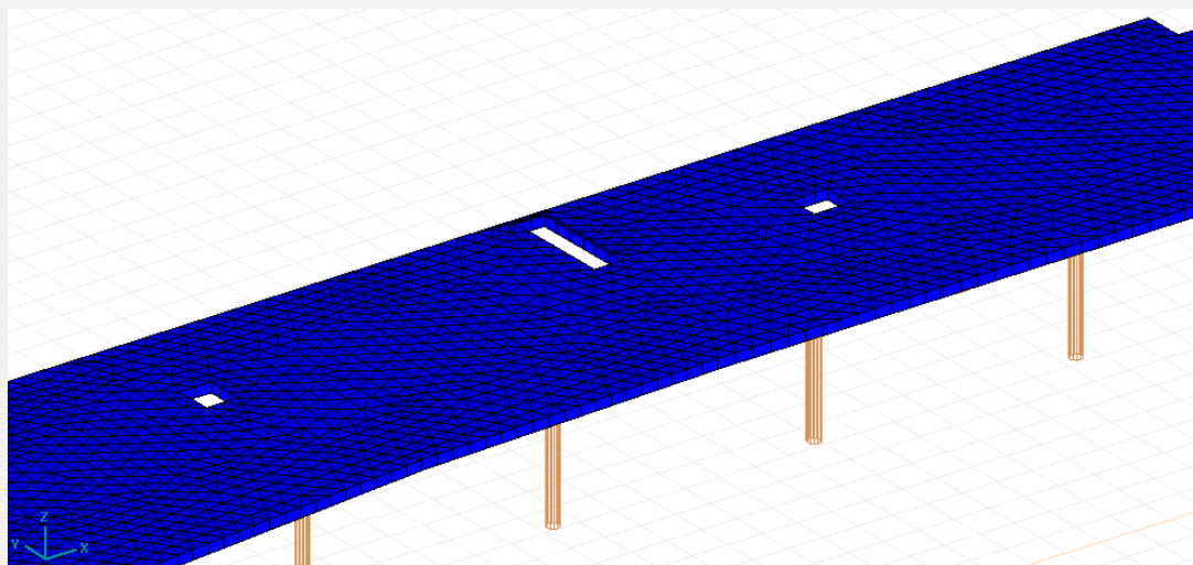
Modelo de cálculo de un forjado (visualización 3D) con algunas aberturas y apoyado en pilares
