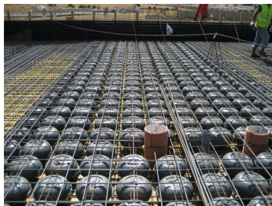
Ejemplos de diversas instalaciones y sistemas de postesado en un forjado COBIAX CLS
