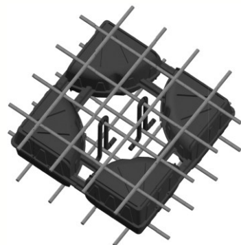
Figura 9 – Posición de los omegas en el interior de la Zona X
