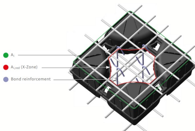
Figura 11 – Ejemplo de refuerzo en la zona X de un forjado COBIAX CLS
