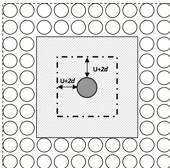
Figura 10 – Zona maciza debido al punzonamiento
