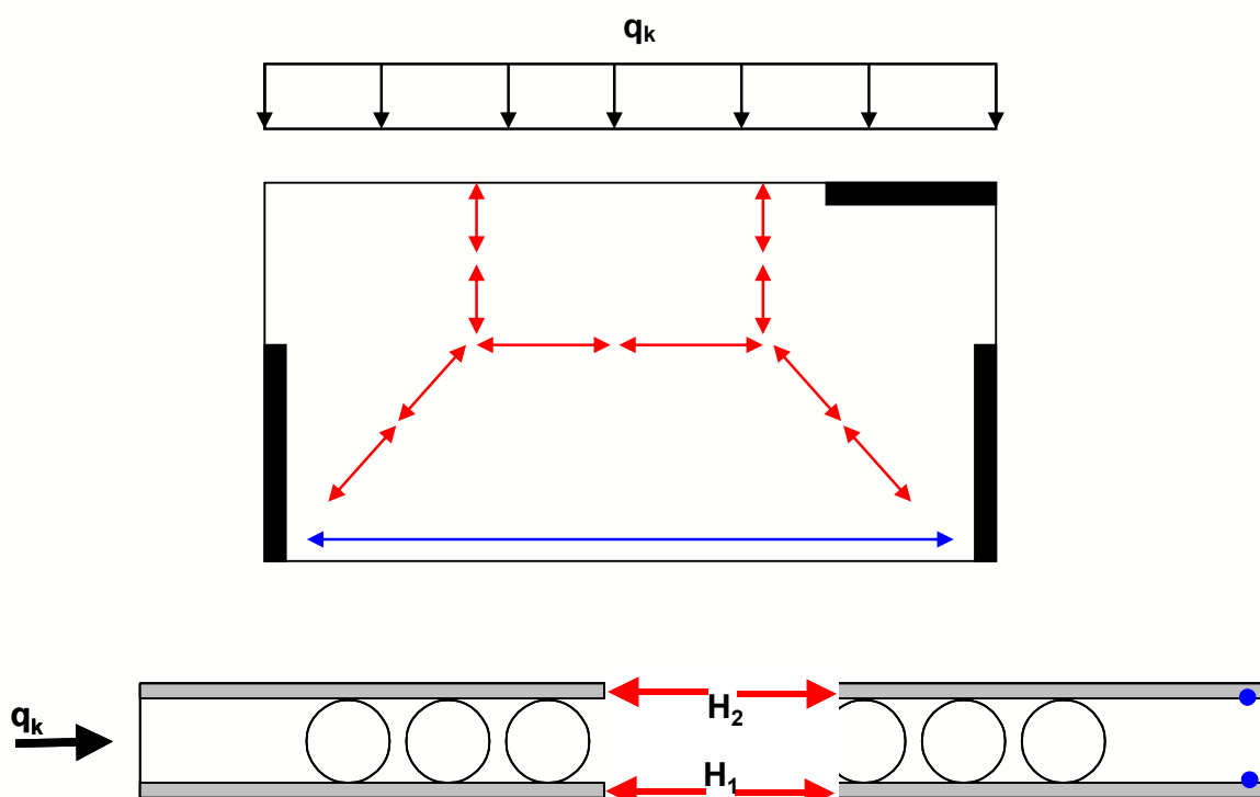
Figura 12 – Comportamiento diafragma del forjado Cobiax
