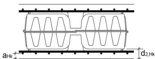
Figura 13 – Distancias relevantes para la resistencia al fuego
