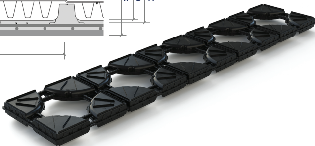
Altura do vazio entre 80mm e 560mm Para lajes de 0,20m a 0,76m
