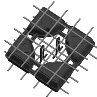
Altura do vazio entre 80mm e 560mm Para lajes de 0,20m a 0,76m
